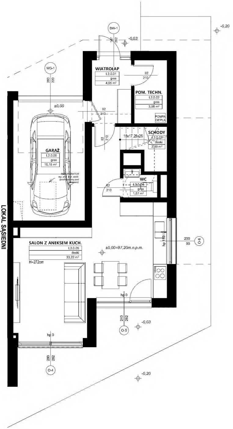
RZUT PARTERU 1:100
